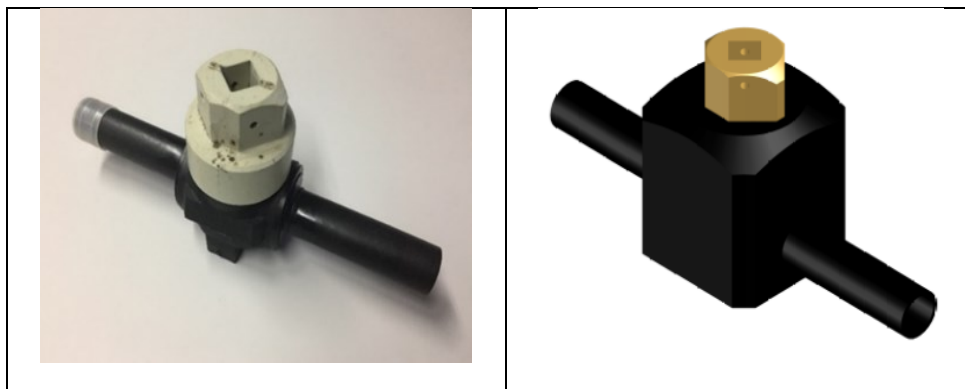
Figura 1 – Exemplos Cabeçote Tipo 1 - Perspectiva
