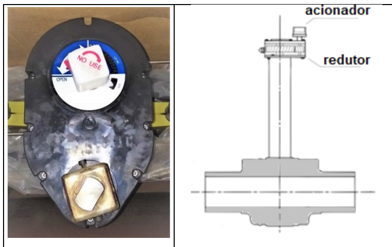
Figura 7 - Exemplo de válvula com acionamento por redutor –
